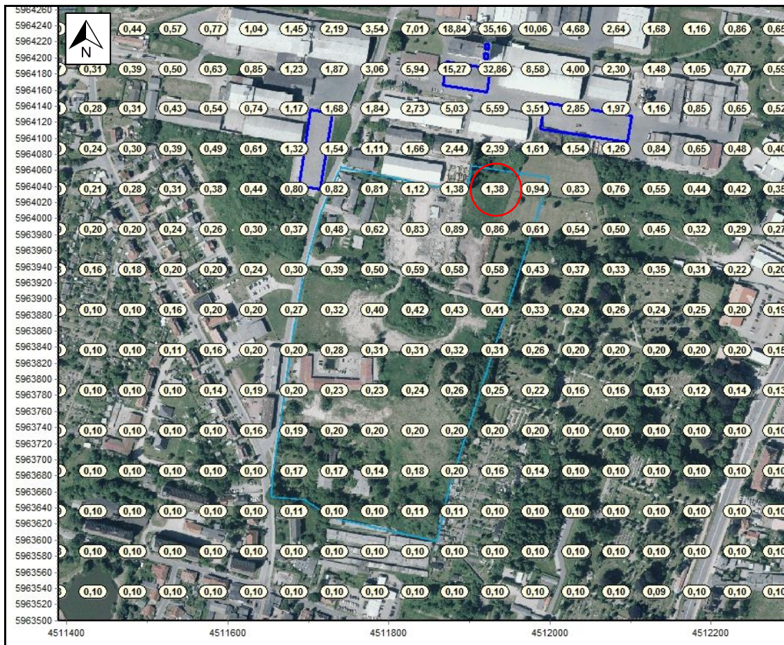
Abb. 8: Flächendarstellung der Tagesmittelwerte für die Konzentration des anlagenbezogenen Feinstaubs der PM 10 -Fraktion im Bereich des Plangebietes (Beurteilungswerte in einem 50 m Raster, errechnet aus einem geschachtelten Rechengitter mit Maschenweiten von 10 m und 20 m), Maßstab 1 : ~8.000
