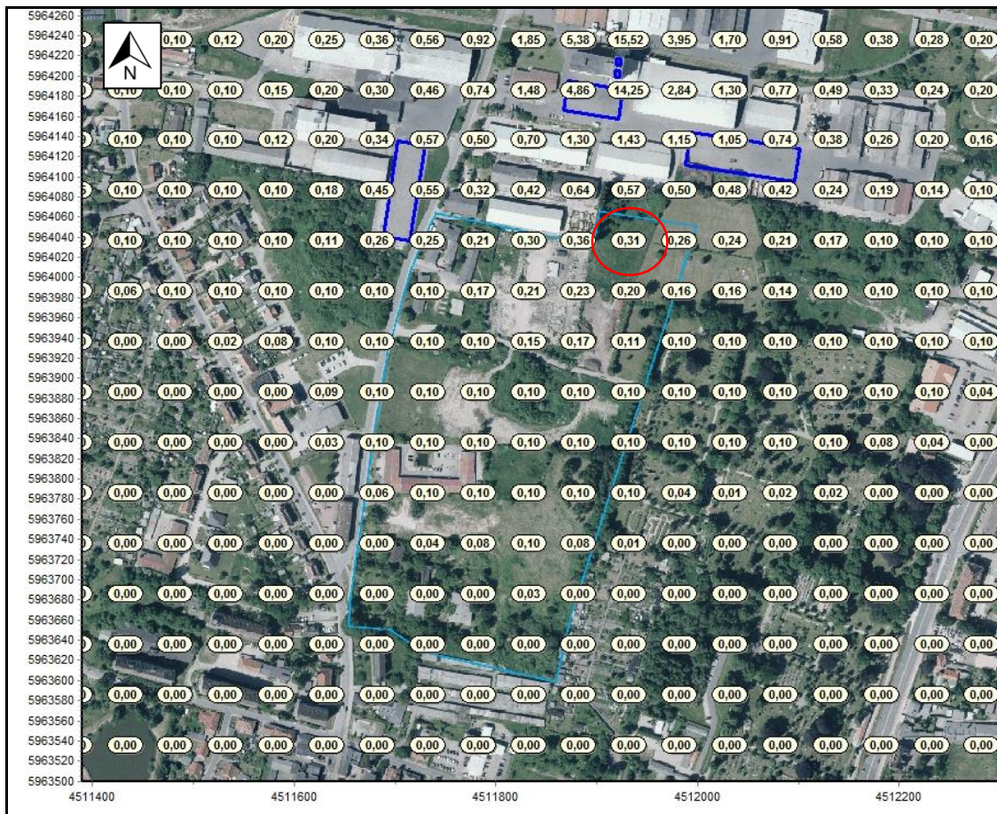
Abb. 7: Beurteilungswerte der Konzentration des anlagenbezogenen Feinstaubs der PM 10 -Fraktion im Plangebiet (Beurteilungswerte in einem 50 m Raster, errechnet aus einem geschachtelten Rechengitter mit Maschenweiten von 10 m und 20 m), Maßstab 1 : ~8.000
