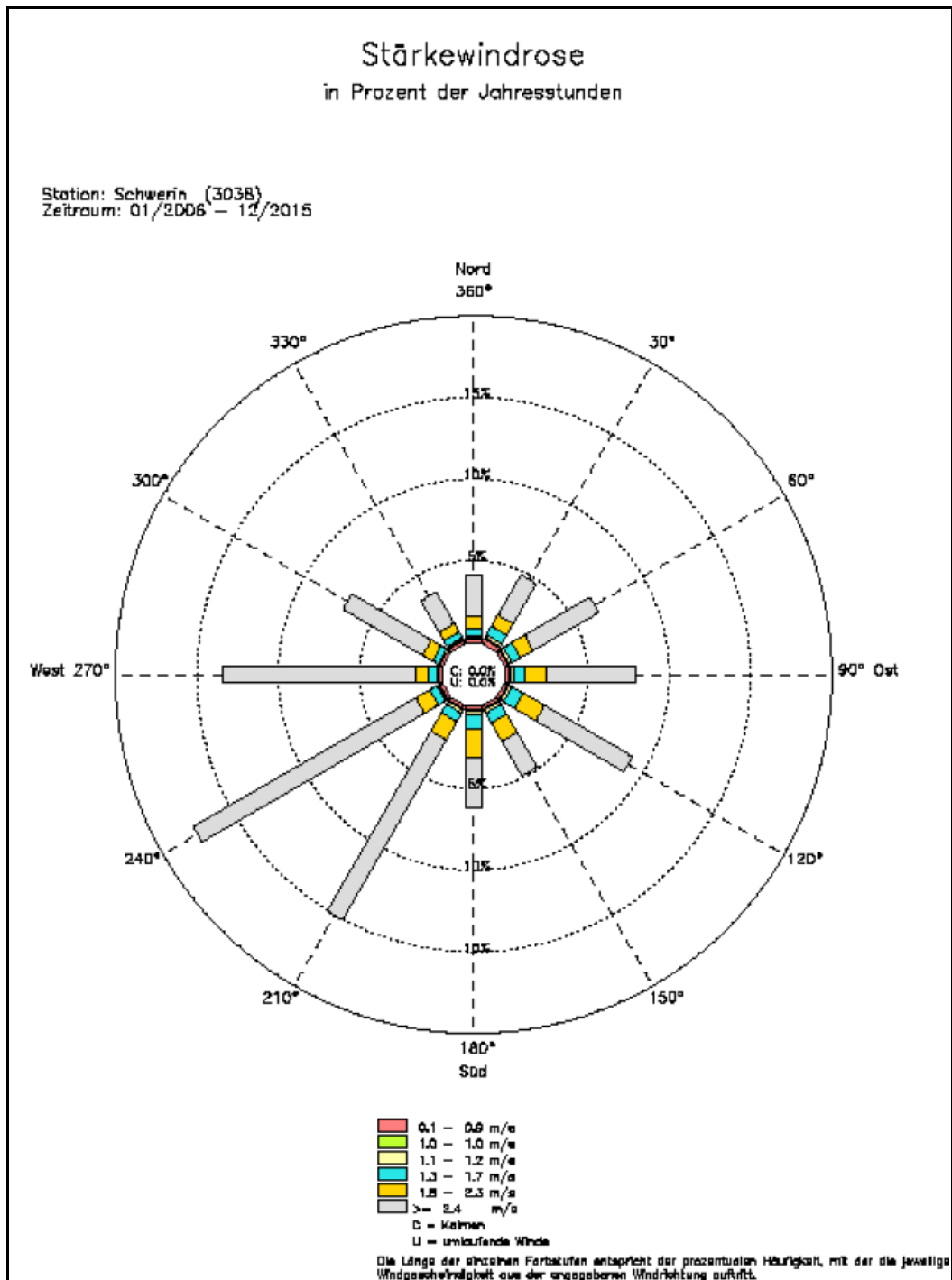
Abb. 5: Darstellung der Stärkewindrose der Windrichtung und der Windgeschwindigkeit in \text{m s}^{-1} am Standort Schwerin (01/2006 – 12/2012)
