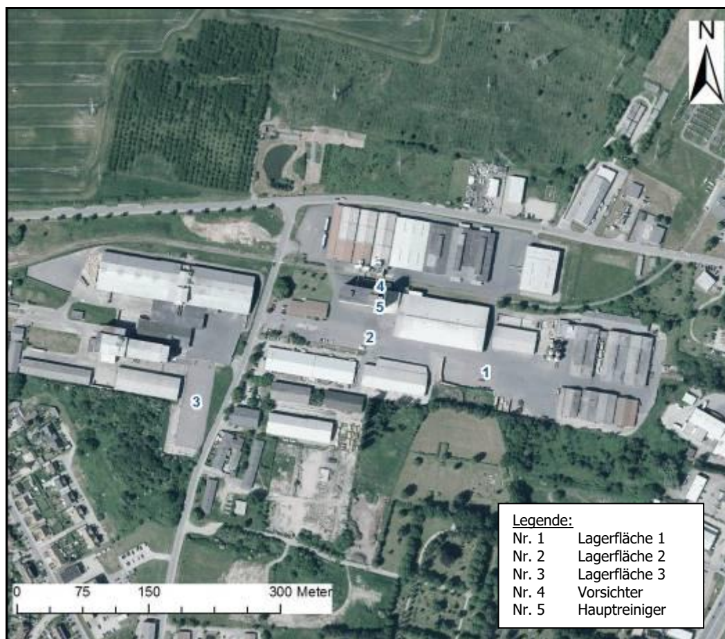
Abb. 3: Lageplan der emissionsrelevanten Quellen auf dem Betriebsgelände der Nordkorn Saaten GmbH.
