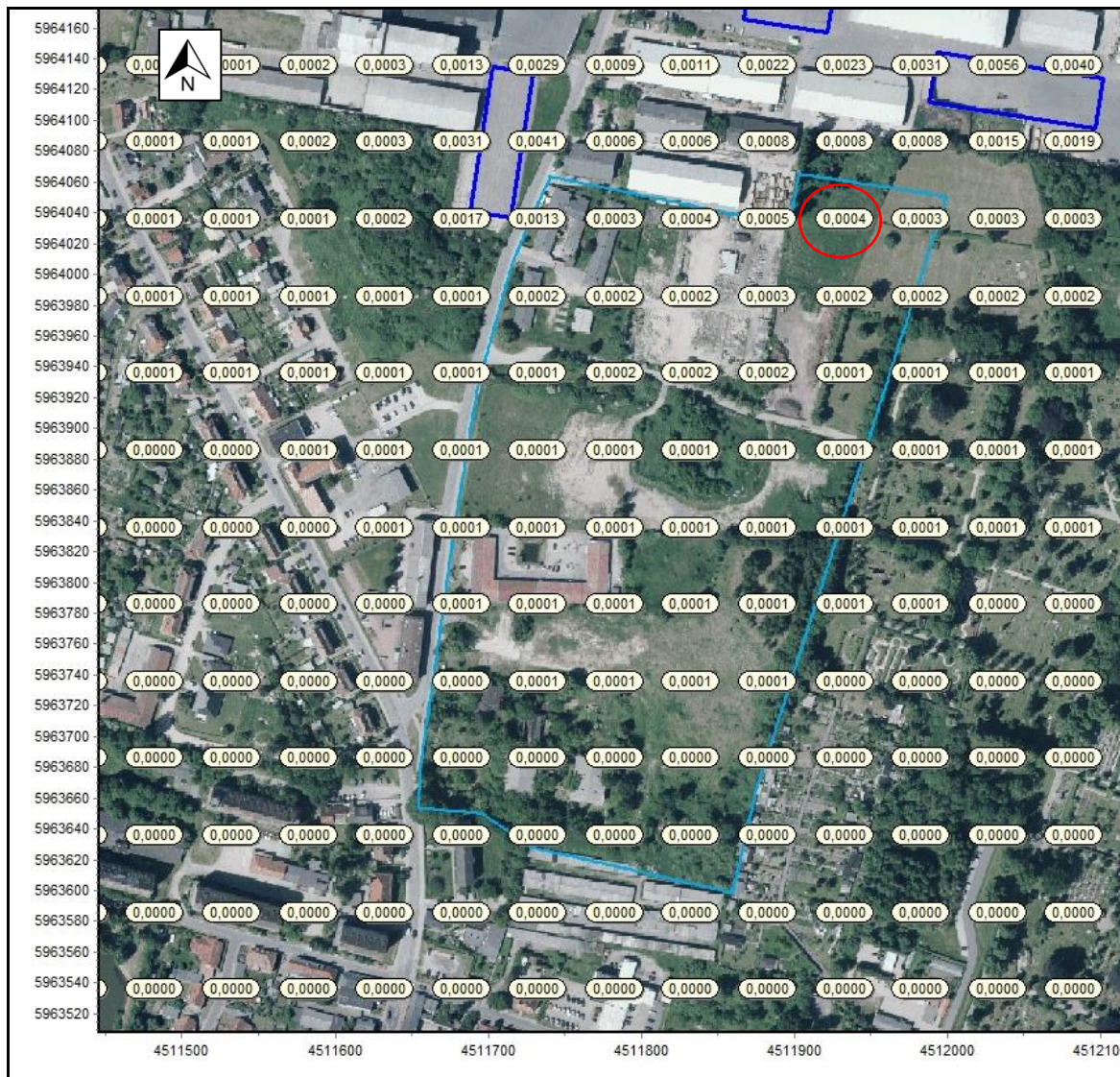
Abb. 9: Flächendarstellung der Zusatzdeposition für den Gesamtstaub in \text{g m}^{-2} \text{d}^{-1} im Jahresmittel im Bereich des Plangebietes (Beurteilungswerte in einem 50 m Raster, errechnet aus einem geschachtelten Rechengitter mit Maschenweiten von 10 m und 20 m), Maßstab 1 : ~4.545
